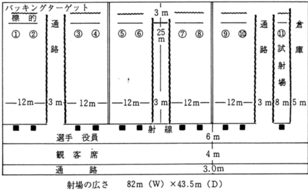
平面図(10グループ, 5 セクション)
