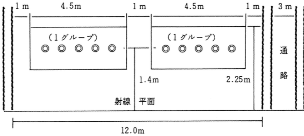
正面図(1 セクション)
