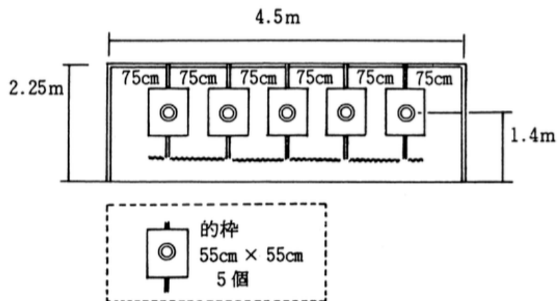
正面図(1グループ, 5ターゲット)
