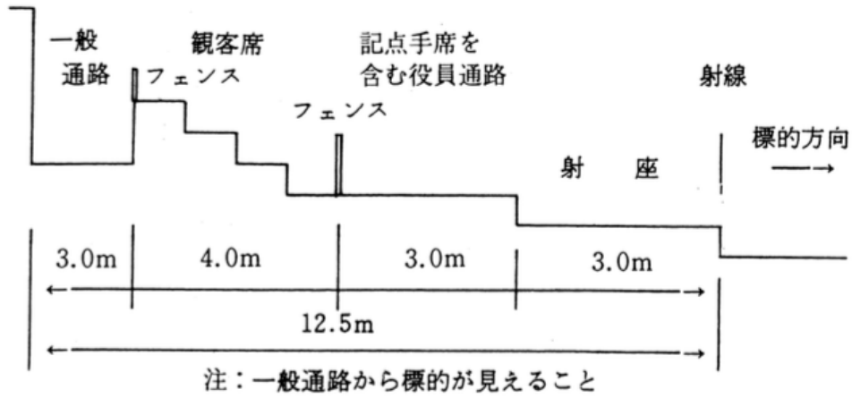
付図—1 射場の断面図
