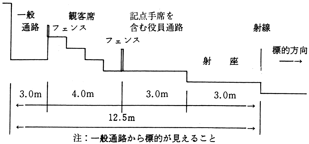
付図—1 射場の断面図
